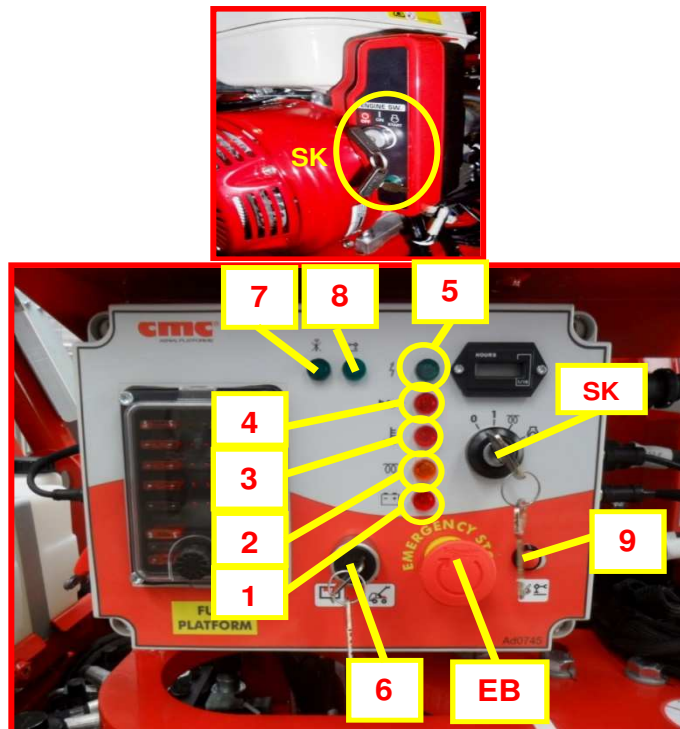
Afbeelding 4: bedieningspost start/stop motor.
